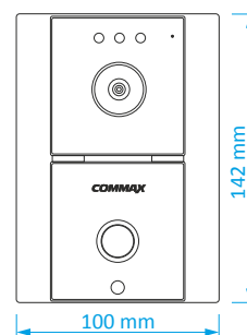
DRC-4L
