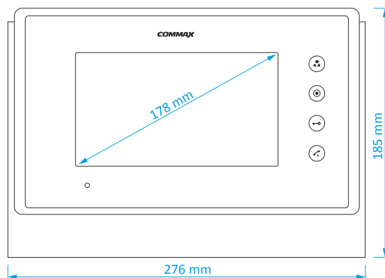
CDV-70UM / CDV-70U
