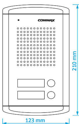
DR-2A2N
