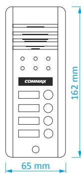
DRC-4DC
