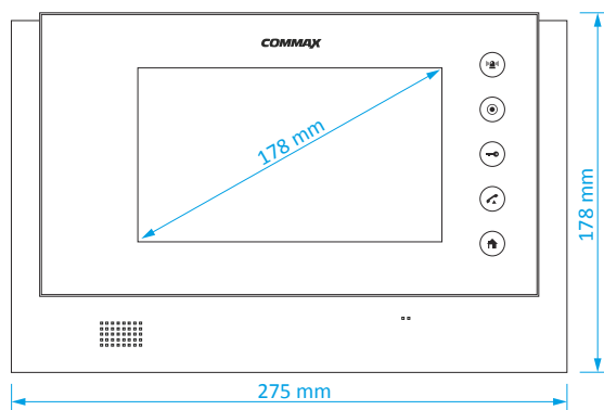
CDV-70UX / CDV-71UM
