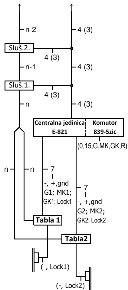
PLAN INSTALACIJE
