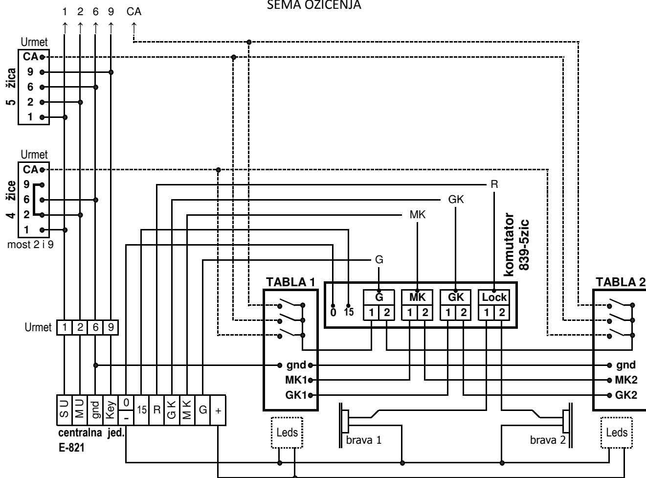
ŠEMA OŽIČENJA
