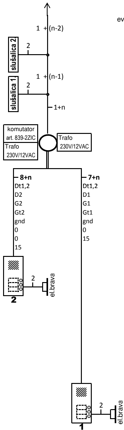
PLAN INSTALACIJE
