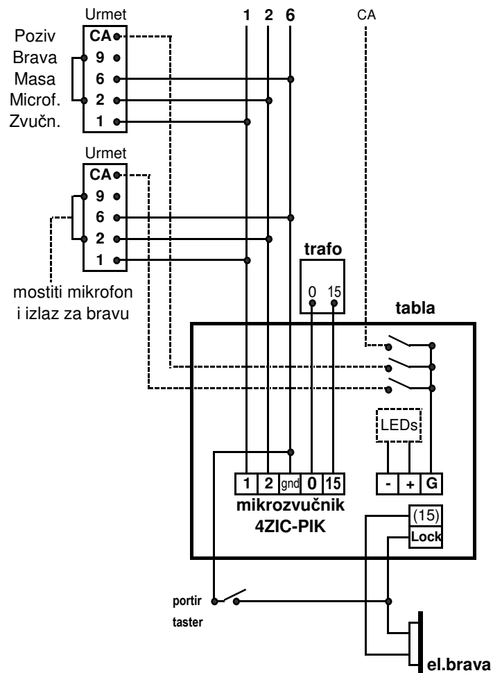
ŠEMA OŽIČENJA
