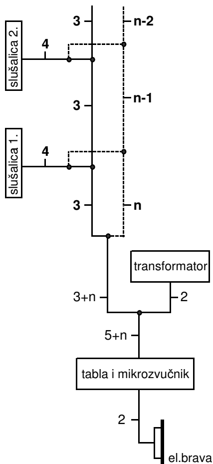
PLAN INSTALACIJE
