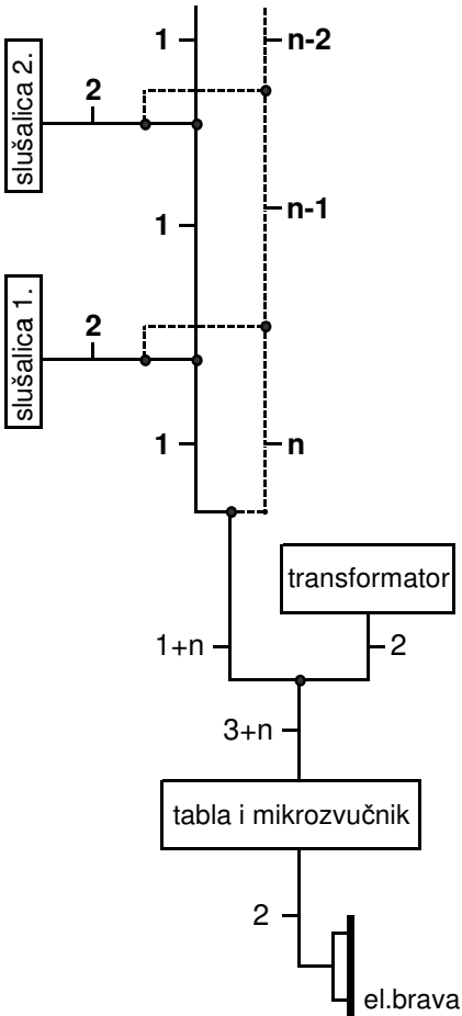
PLAN INSTALACIJE
