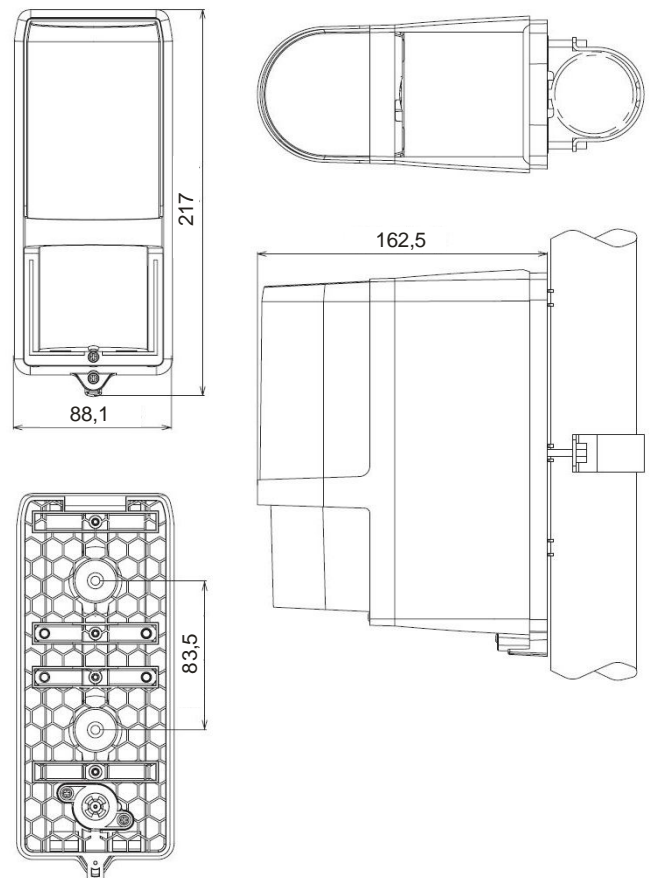
Fig. 10 Unit dimensions
